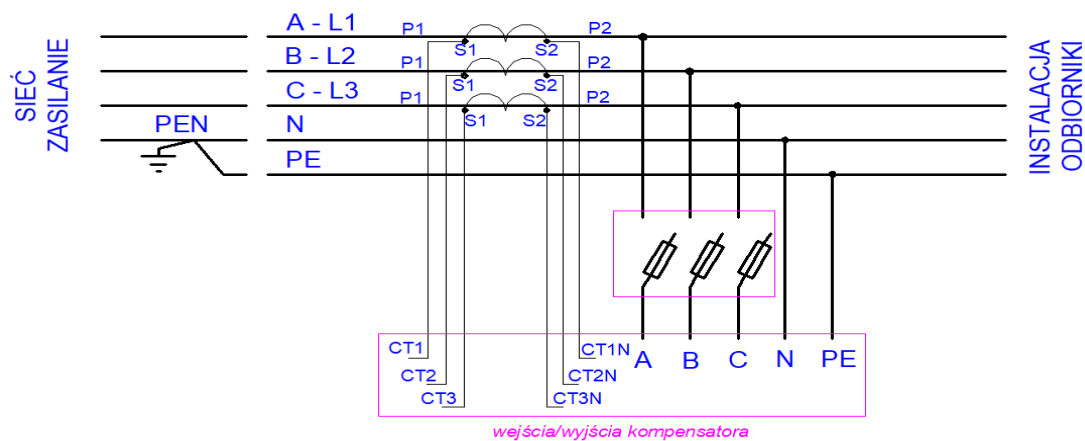
Rysunek 3. Układ podłączenia przekładników od strony sieci.
