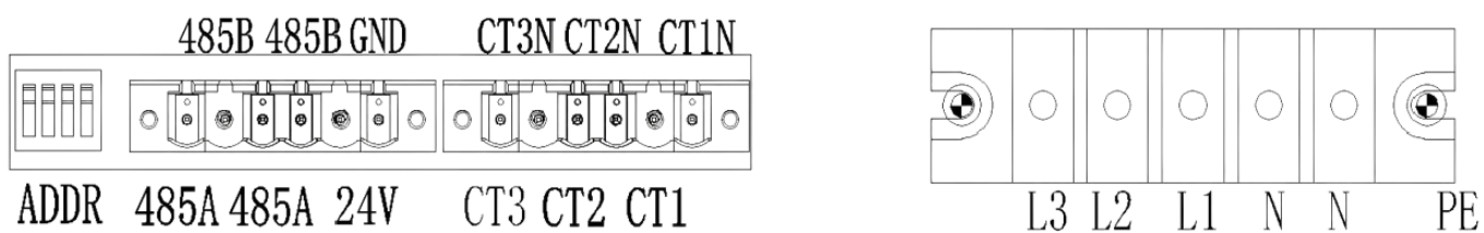
Rysunek 2. Widok złączy oraz wejść kompensatora.
