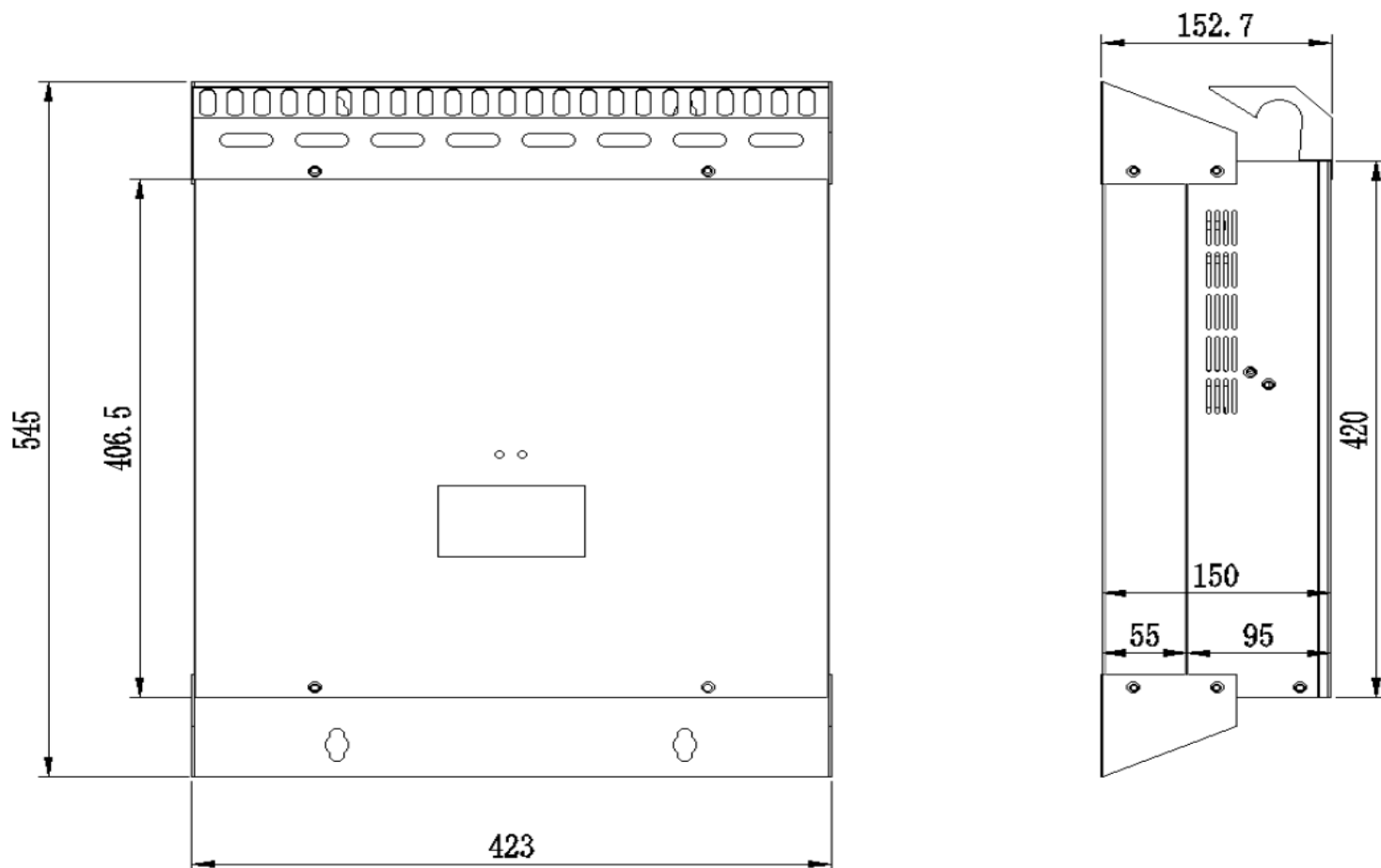
Rysunek 1. Wymiary kompensatora REACTO mocy 10kVar
