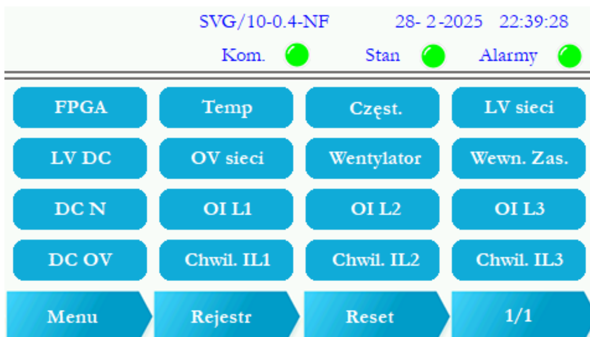
Ekran 17. Karta alarmów.
