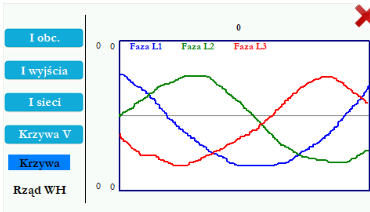
Ekran 19. Przebiegi prądów.
