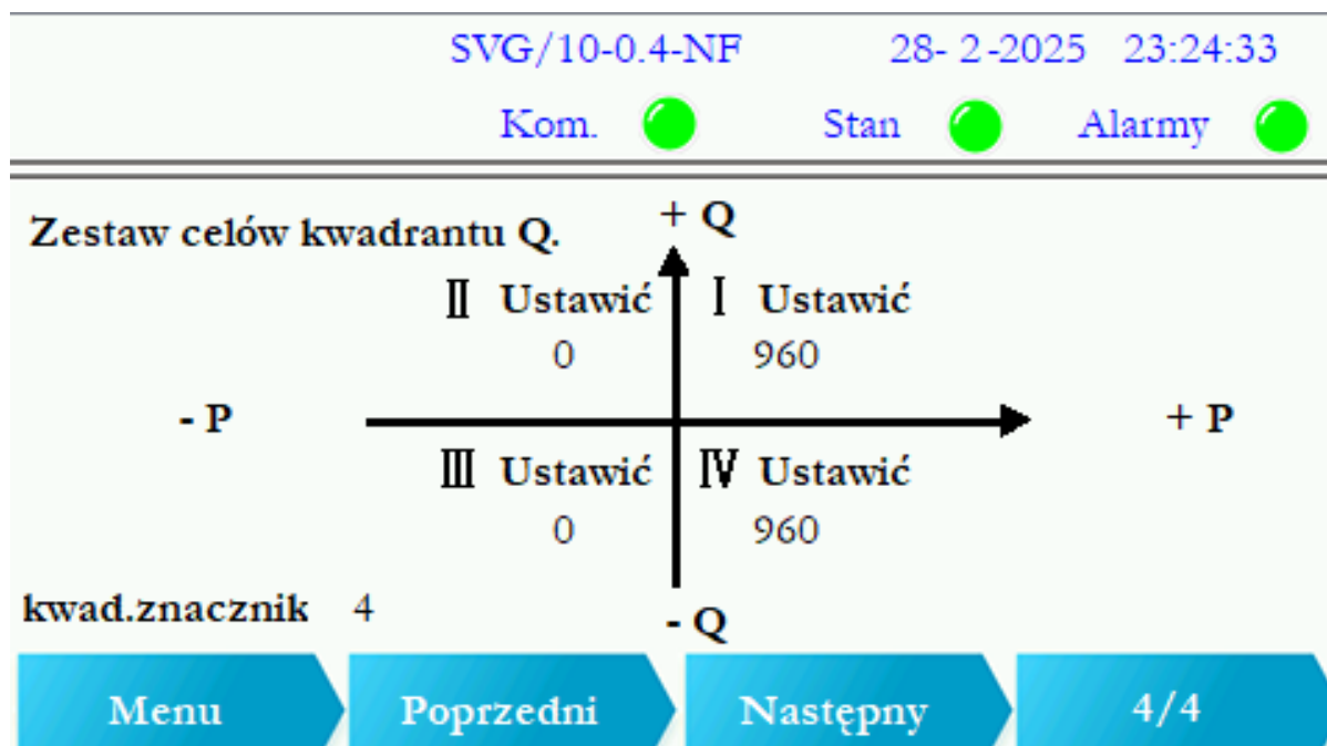
Ekran 9. Ustawienia 4/4 - cele kompensacji.
