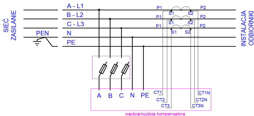
Rysunek 4. Układ podłączenia przekładników od strony instalacji.
